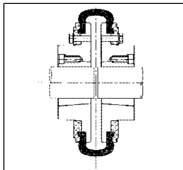
SIZES F70-250
